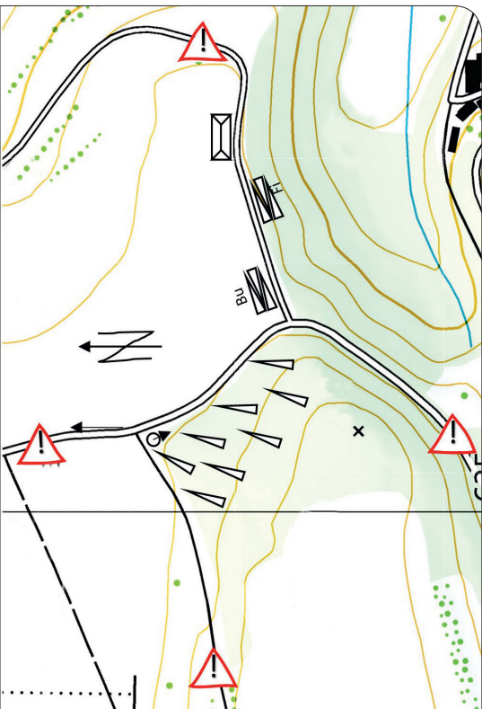
Lo schizzo di taglio fornisce informazioni sulle aree di stoccaggio, la direzione di esbosco, la direzione di taglio e di abbattimento e la segnaletica necessaria.
